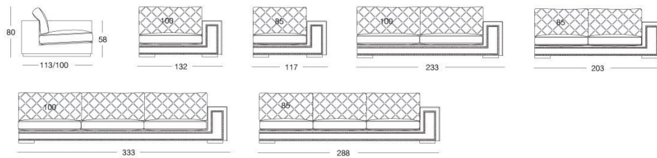
Terminali Dx / End unit R.H. / Боковые секции П
